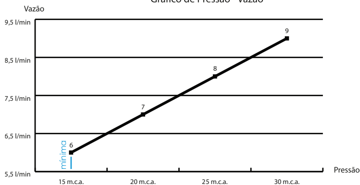
Gráfico de Pressão - Vazão
