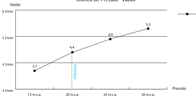
Gráfico de Pressão - Vazão
