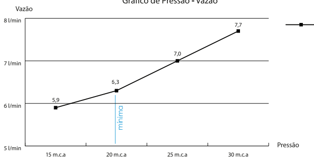
Gráfico de Pressão - Vazão
