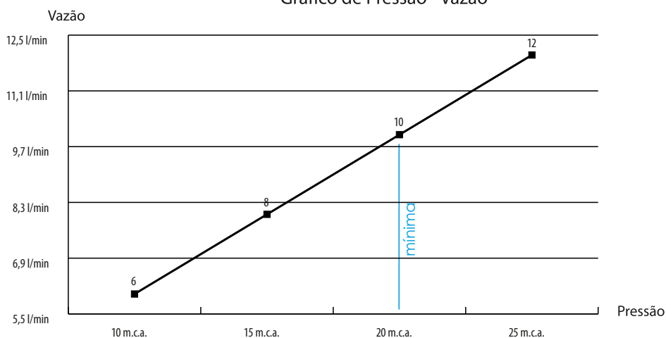
Gráfico de Pressão - Vazão
